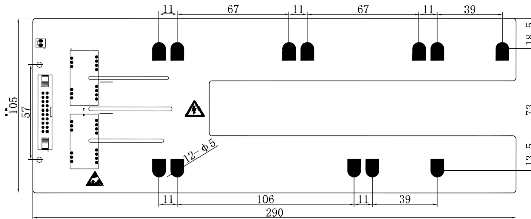
图2 产品结构尺寸
