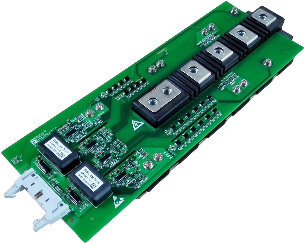
图 1 4QP0115T12-3L-D 产品展示
